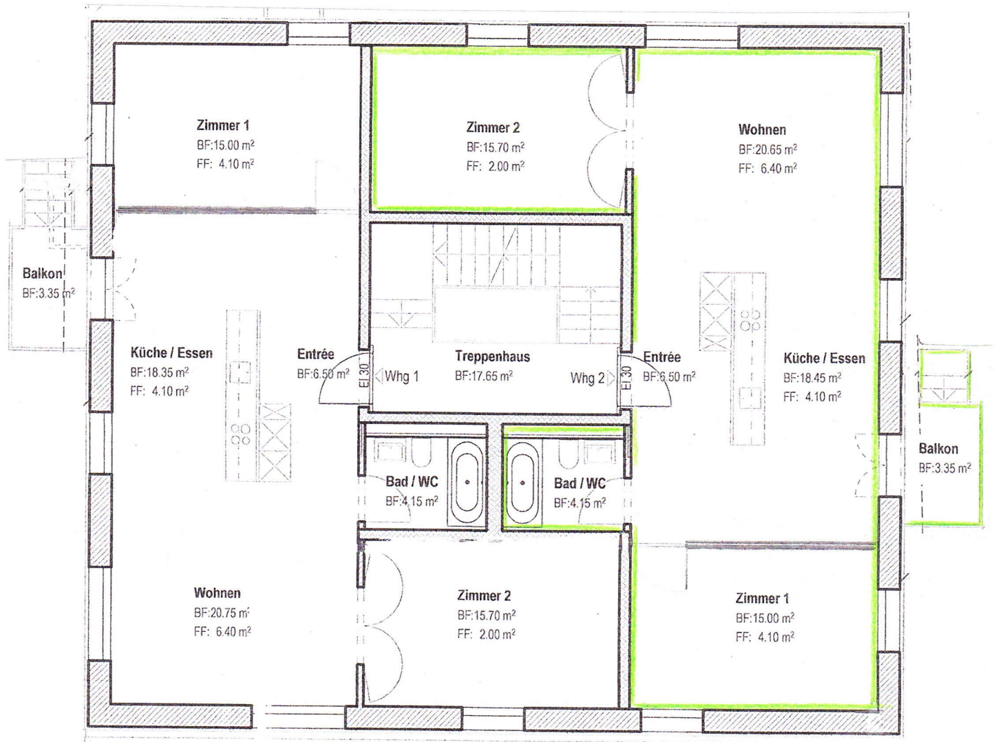
Wohnung 2 = 3.5 Zimmer-Wohnung Balkon mit Treppe zu Sitzplatz und Gartenanteil, Ausrichtung Nordwesten NGF Total 80.45 m 2
